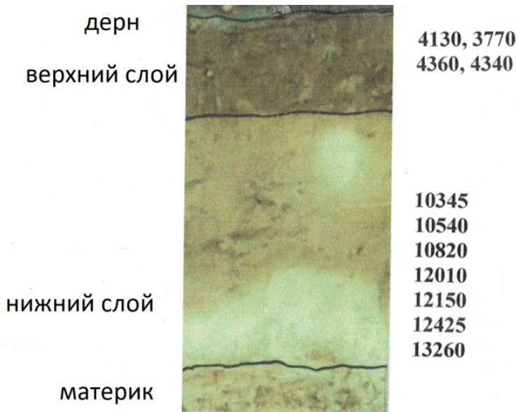
Илл. 2. Разрез культурных напластований поселения Хумми (верхний слой мощностью 20–24 см, нижний слой — 40–45 см)
